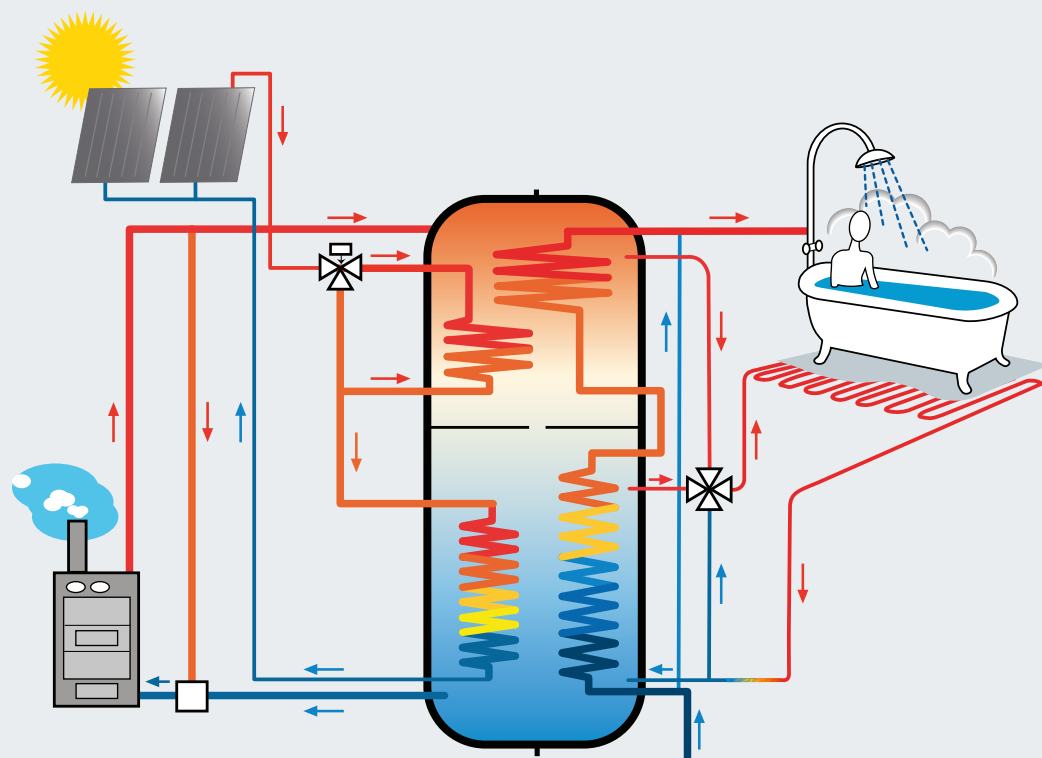
AKVA SOLAR PLUS med solfångare och vedpanna
